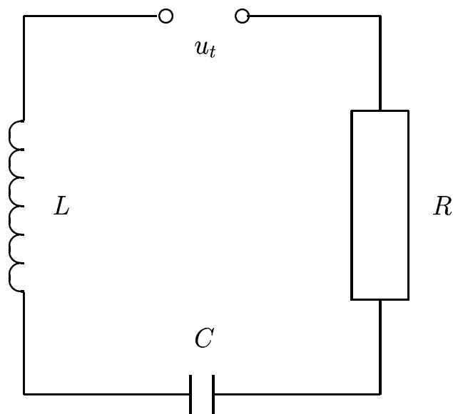
Рис. 2.5. Электрическая цепь.
