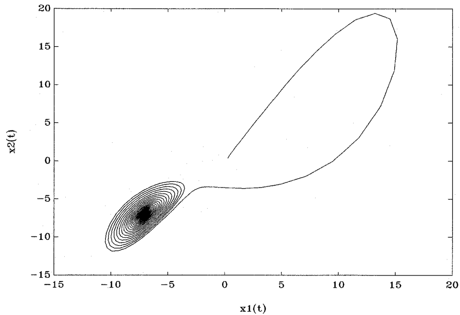
Рис.14.3. Фазовый портрет системы уравнений Лоренца при b = 8/3 , a = 10 , r = 19.8 .
