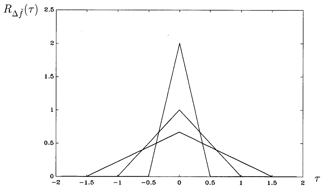
Рис.1.1. График семейства функций R_{\Delta \tilde{f}}(\tau) .
