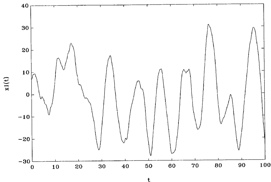
Рис.13.6. Моделирование солнечной активности при \lambda = 0.07 , \sqrt{a_2} = 0.5661 , c = 5.08 .
