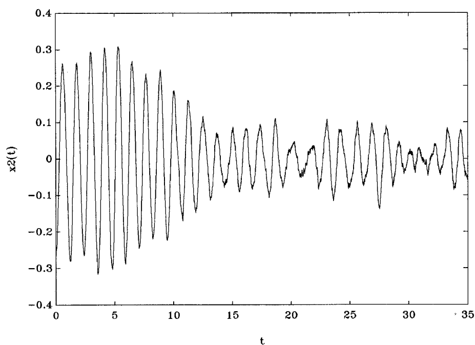
Рис.13.3. Моделирование чандлеровских колебаний при \lambda = 0.06 , a = 0.035 , \omega = 5.274 .
