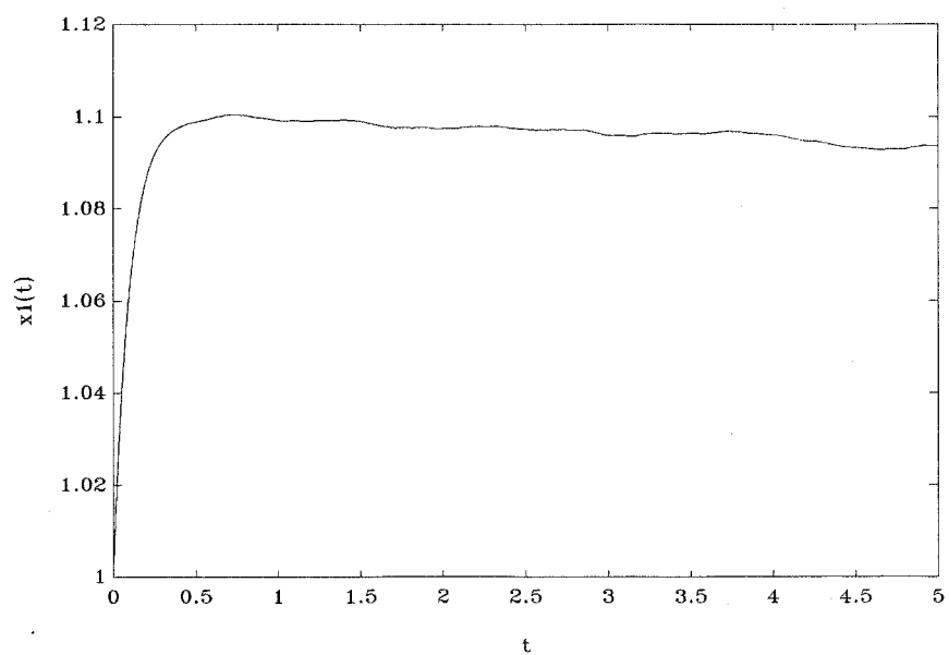
Рис.13.8. Моделирование лагранжевой динамики частицы жидкости при T = 0.1 , \sigma = 0.02 , \Delta = 0.002 .
