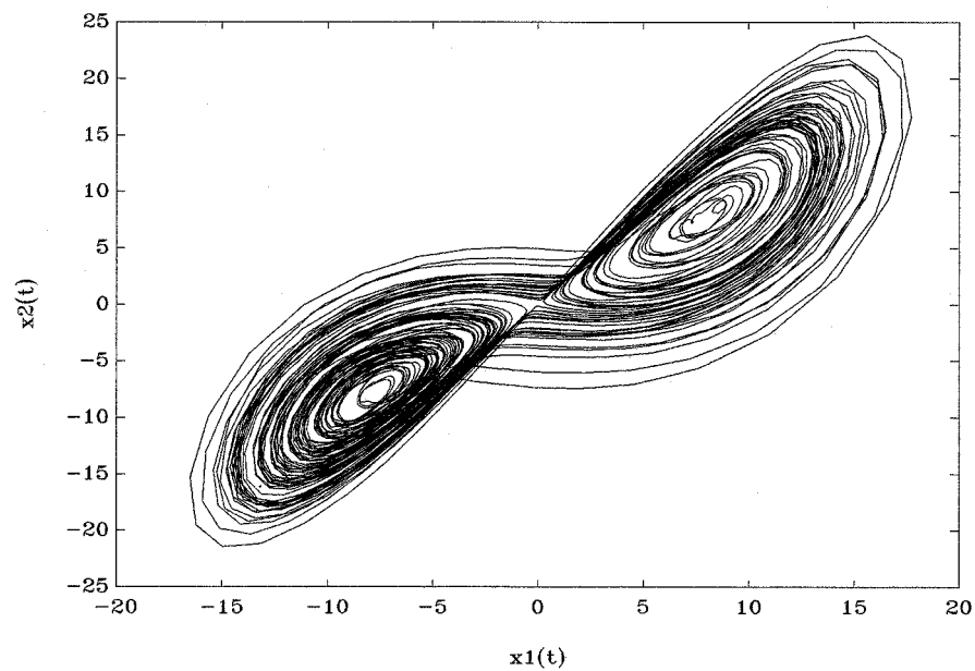
Рис.14.14. Фазовый портрет системы уравнений Лоренца со стохастическим возмущением при b = 8/3 , a = 10 , r = 24.3 , c = 4.0 .
