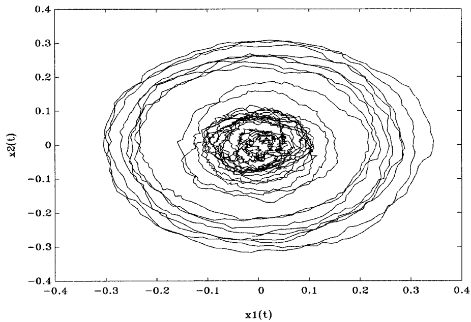
Рис.13.4. Чандлеровские колебания. Фазовый портрет при \lambda = 0.06 , a = 0.035 , \omega = 5.274 .
